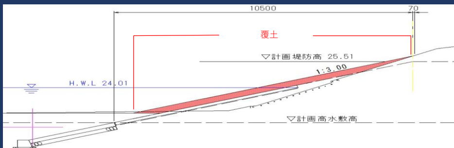
施工図面 （赤・・・覆土箇所）
