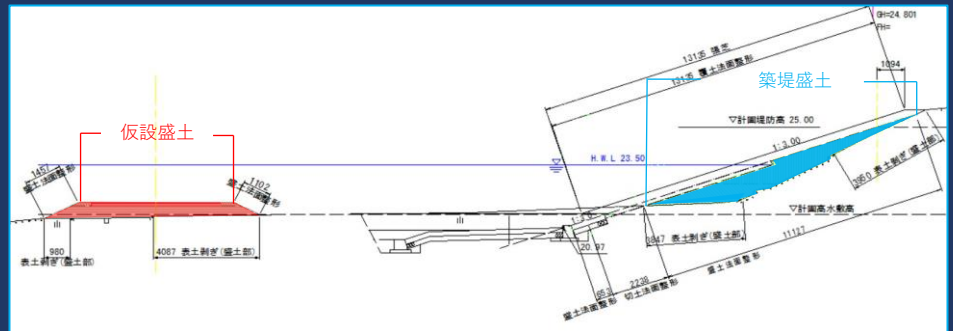
施工状況 (赤・・・仮設盛土箇所 青・・・築堤盛土箇所)
