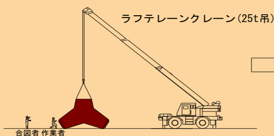
1. 下部型枠組立
