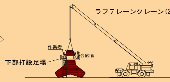
3. 上部型枠組立
