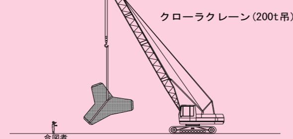
8. 仮置
