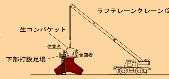
2. 下部コンクリート打設
