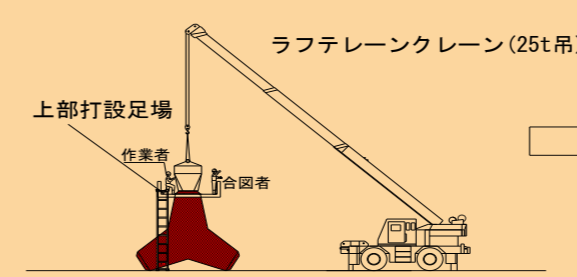
4. 上部コンクリート打設
