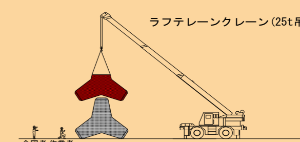
5. 型枠脱型
